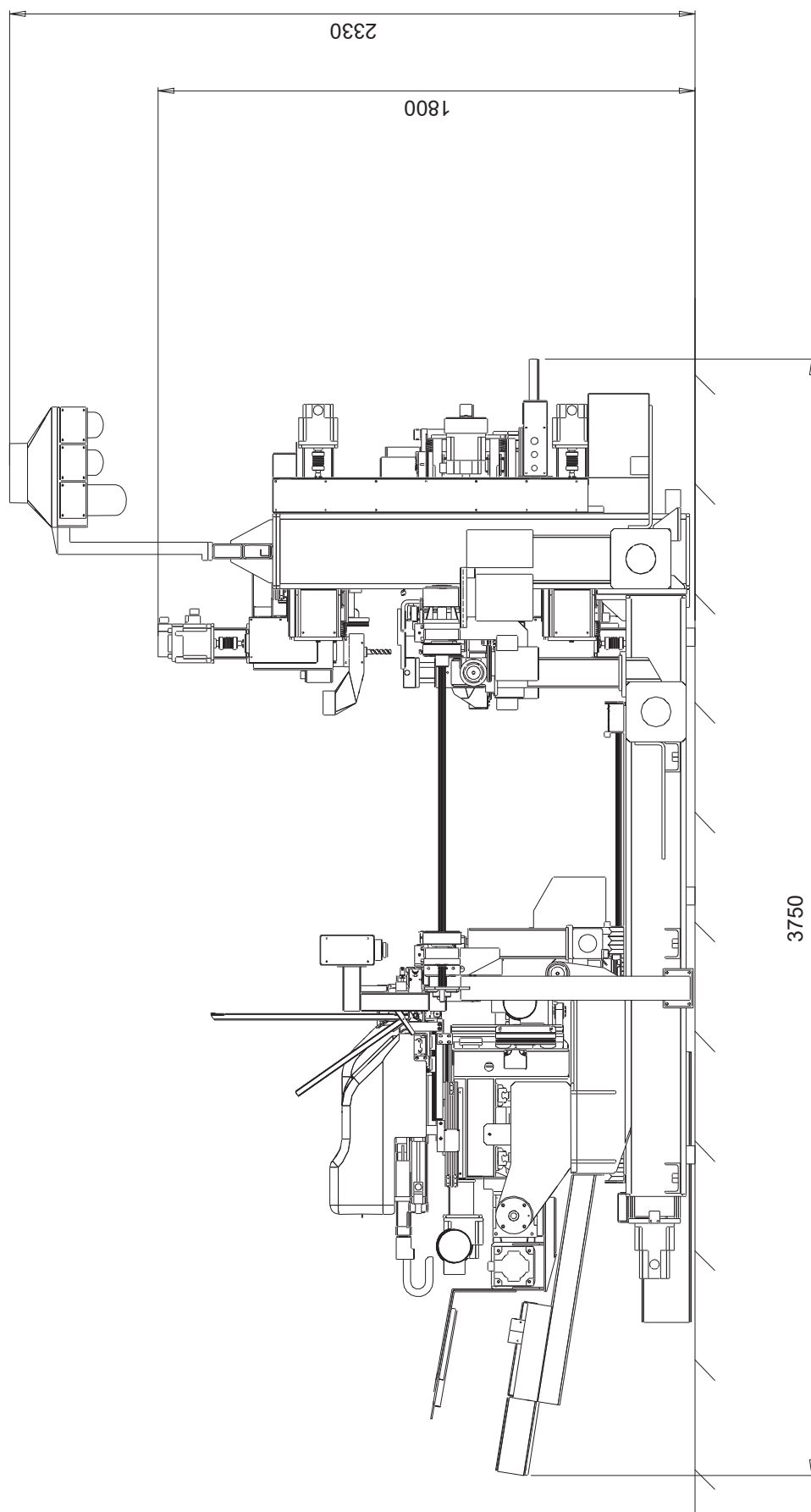
VISTA LATERALE DELLA MACCHINA CON QUOTE D'INGOMBRO
